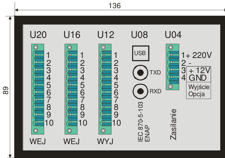
Rys 2. Widok urządzenia CSA-12 od strony wyprowadzeń
