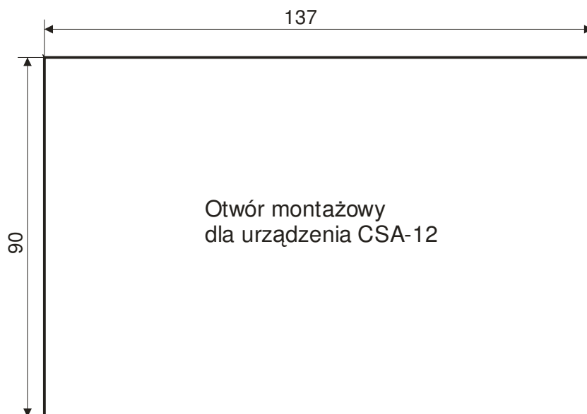
Rys 3. Otwór montażowy urządzenia CSA-12.
