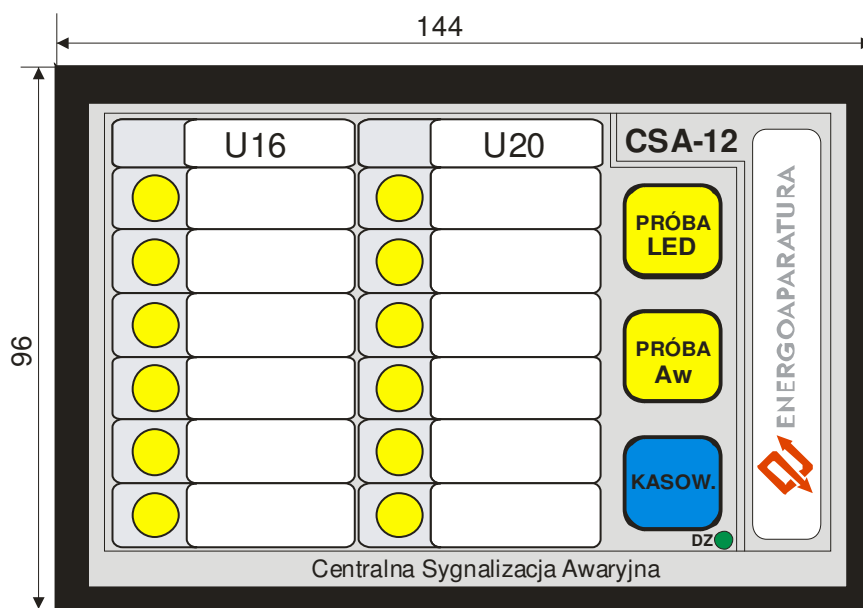
Wymiary zewnętrzne frontu urządzenia
