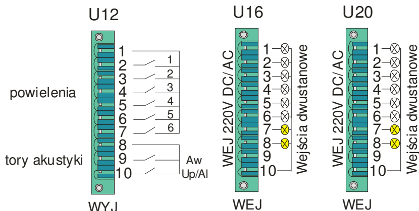
Rys 3. Graficzny opis wyjść wejść.
