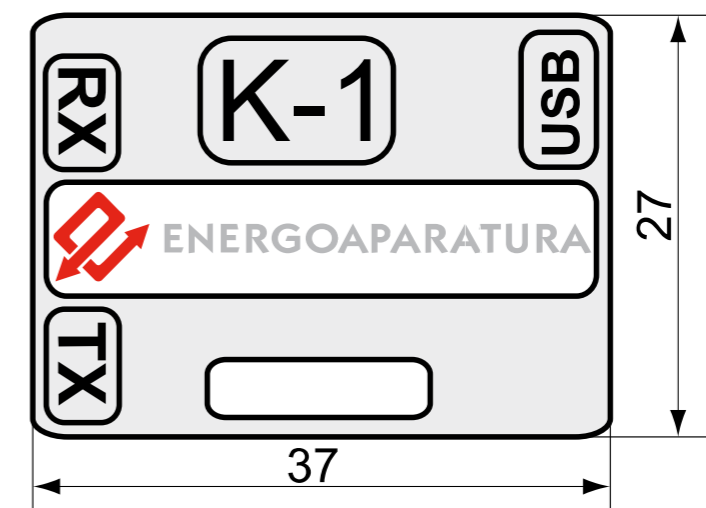
Rys. 1. Rysunek techniczny konwertera K-1
